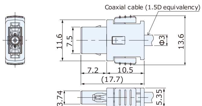
Plug : CRC9001-7701F
