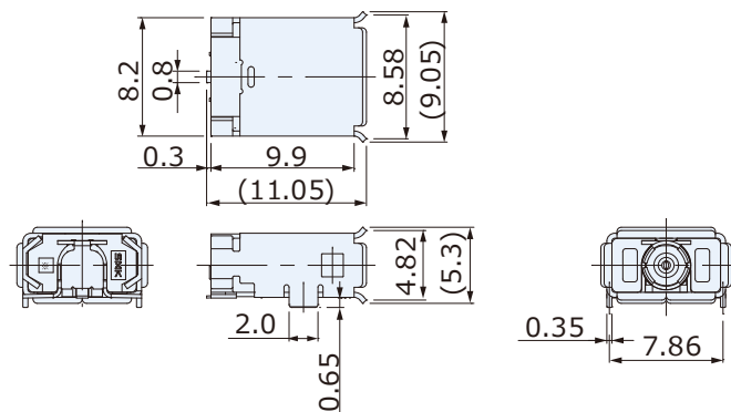
Receptacle : CRS5001-4701F
